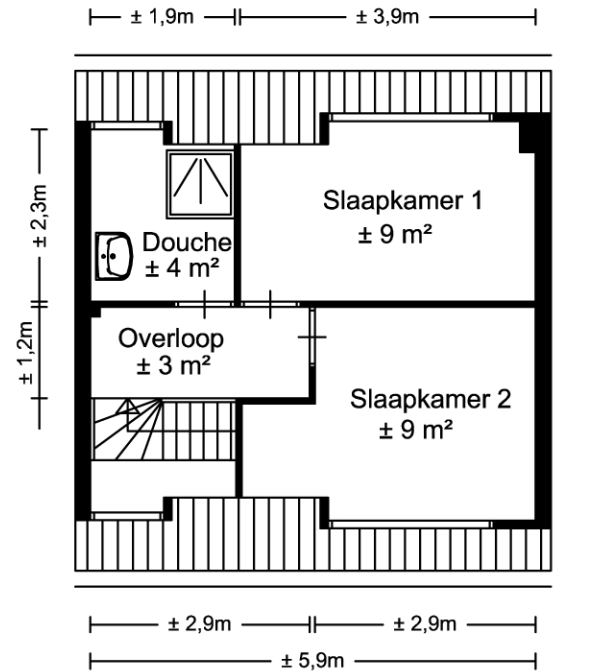
Verdieping
